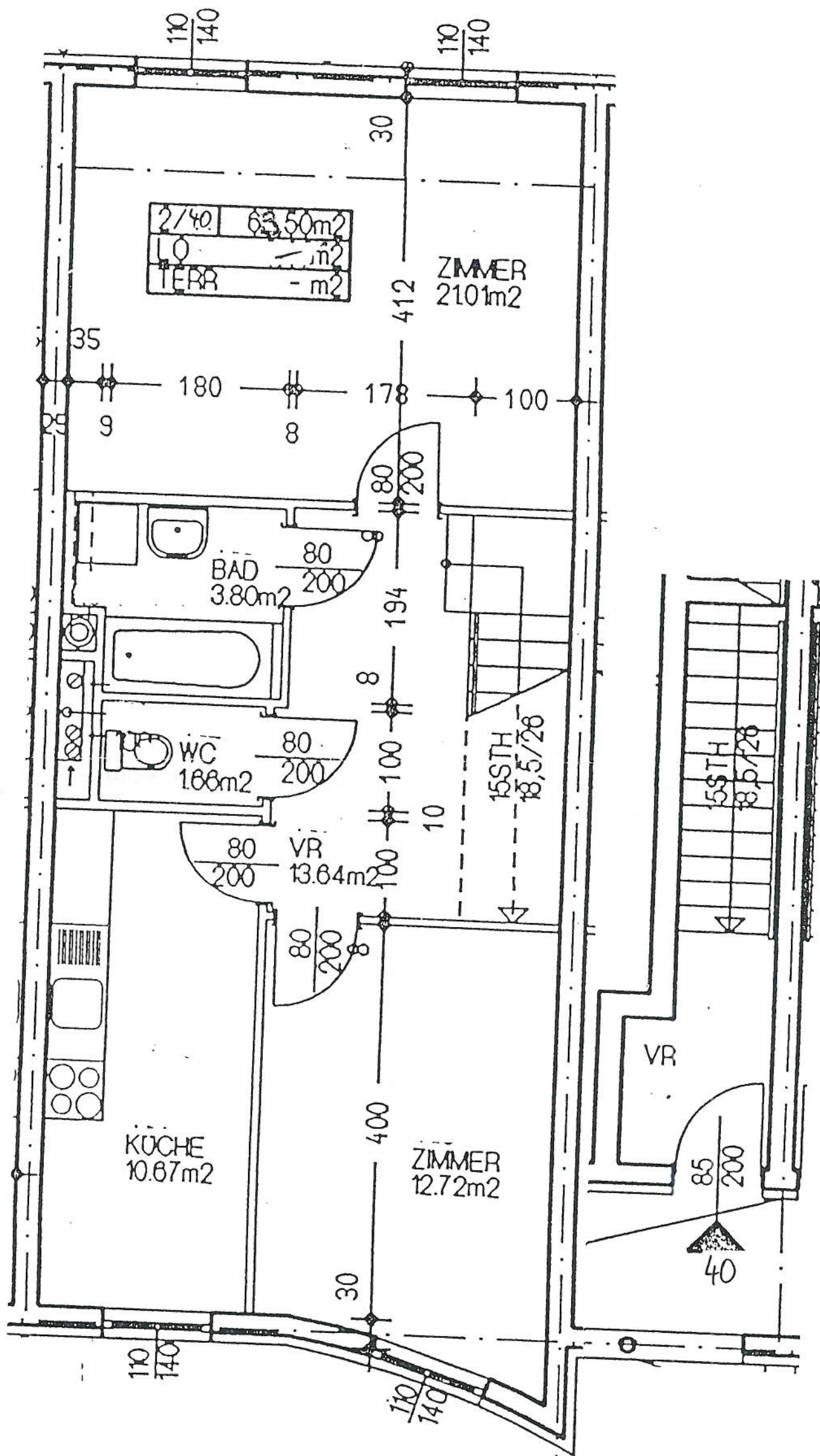
GRUNDRISS 3.OG 1:50
