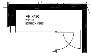
GRUNDRISSAUSSCHNITT ERDGESCHOSS
